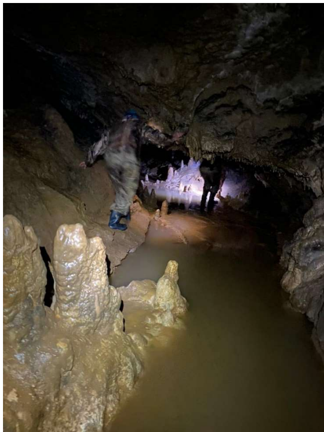
Нижний карстовый зал, ручей
