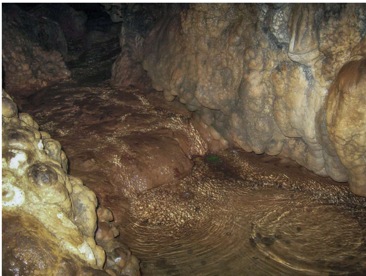
Пещерная река Лозовушка
