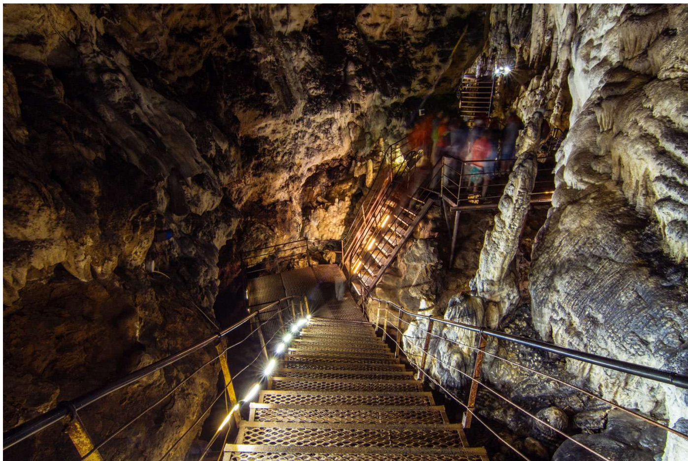
Пещера хорошо освещен и оборудована надежными ступенями и перилами
