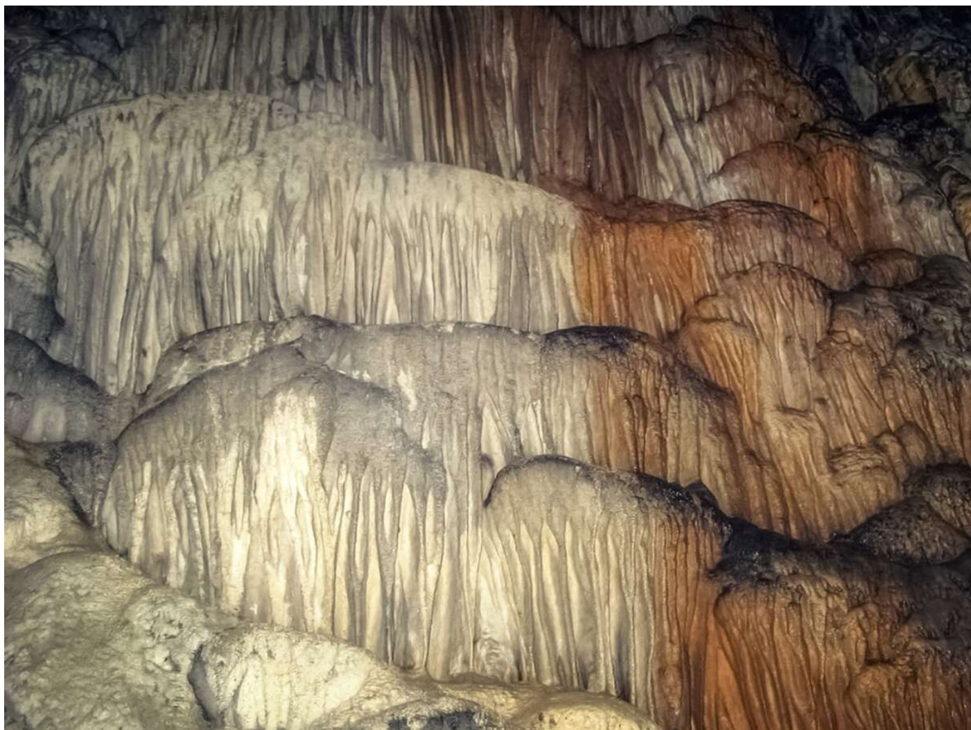
" Органный зал" пещеры. Здесь натечные образования окрашены в разные цвета.
